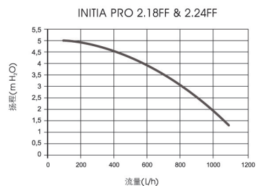
扬程曲线图
